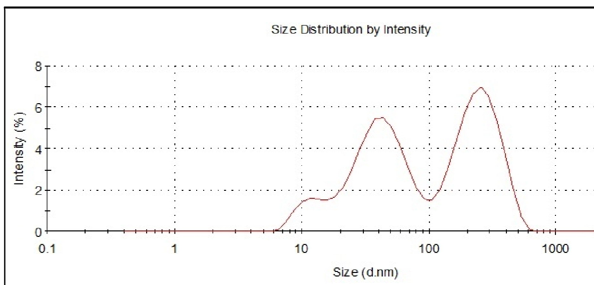
شکل 2 هیستوگرام توزیع اندازه نانو ذره نقره Z-Average(d-nm)=102.3
