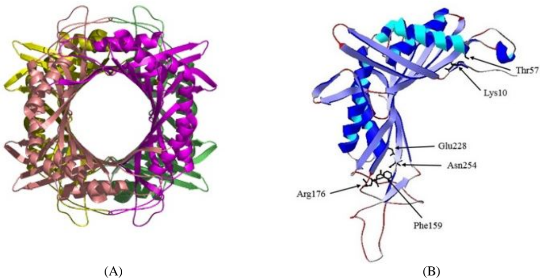
شکل 2 ساختار آنزیم اوریکاز از اسپیریلوس فلاووس. (A) ساختار هوموتراپمر آنزیم اوریکاز (B) ساختار یک زیر واحد آنزیم اوریکاز و رزیدوهای درگیر در جایگاه فعال را نشان می‌دهد. فایل اطلاعات ساختاری آنزیم اوریکاز با کد 4OQC از سایت www.pdb.org گرفته شده است. این ساختار با استفاده از نرم‌افزار SPDBV تهیه شد. جایگاه فعال شامل لیزین 10، ترئونین 57، فنیل آلانین 159، آرژینین 176، گلوتامیک اسید 228 و آسپاراژین 254 می‌باشد.
